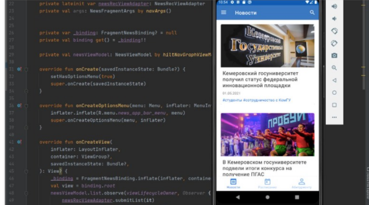
Фрагмент кода и результат работы кода на экране.
